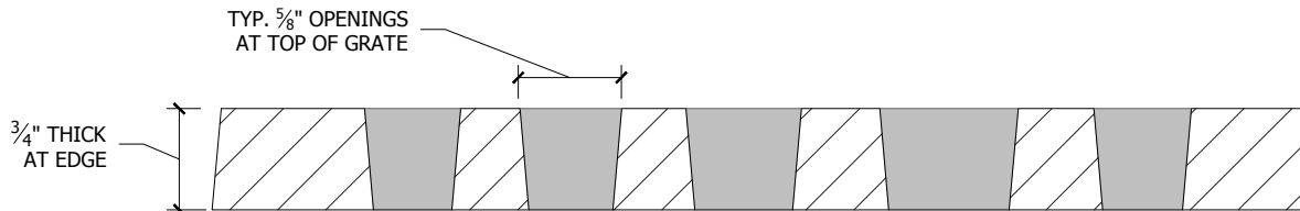
Section A-A'
